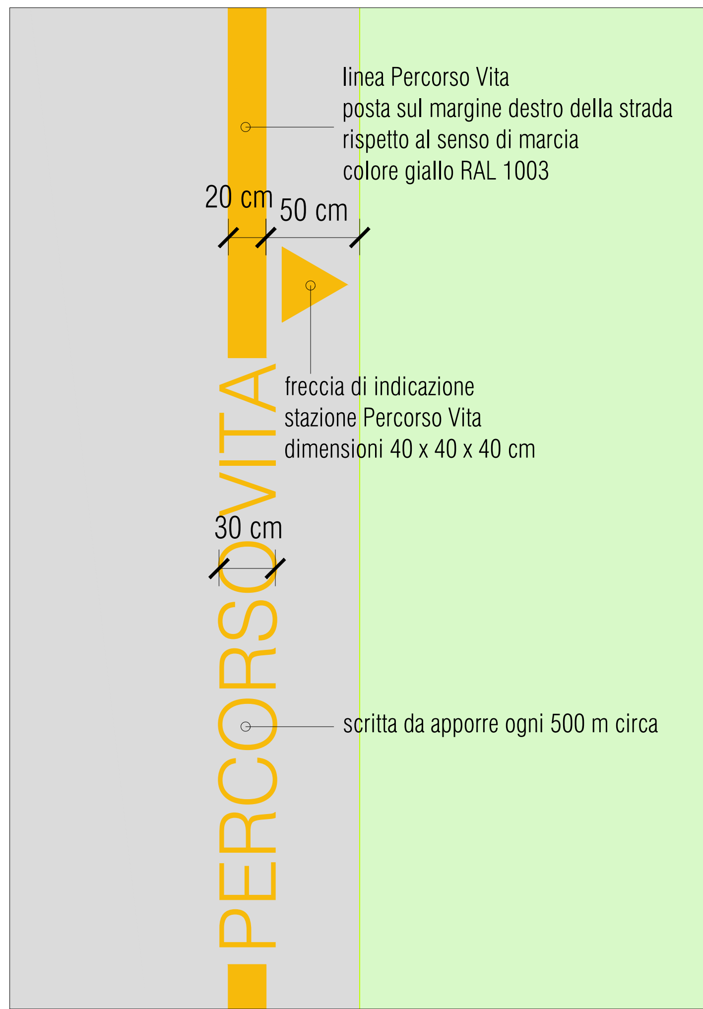
ESEMPIO DI DERMACAZIONE CON VERNICE GIALLA RAL 1003 DEL PERCORSO VITA CON INDICAZIONE DELLE STAZIONI - scala 1:20
